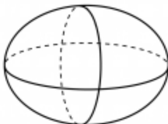
ovoid
